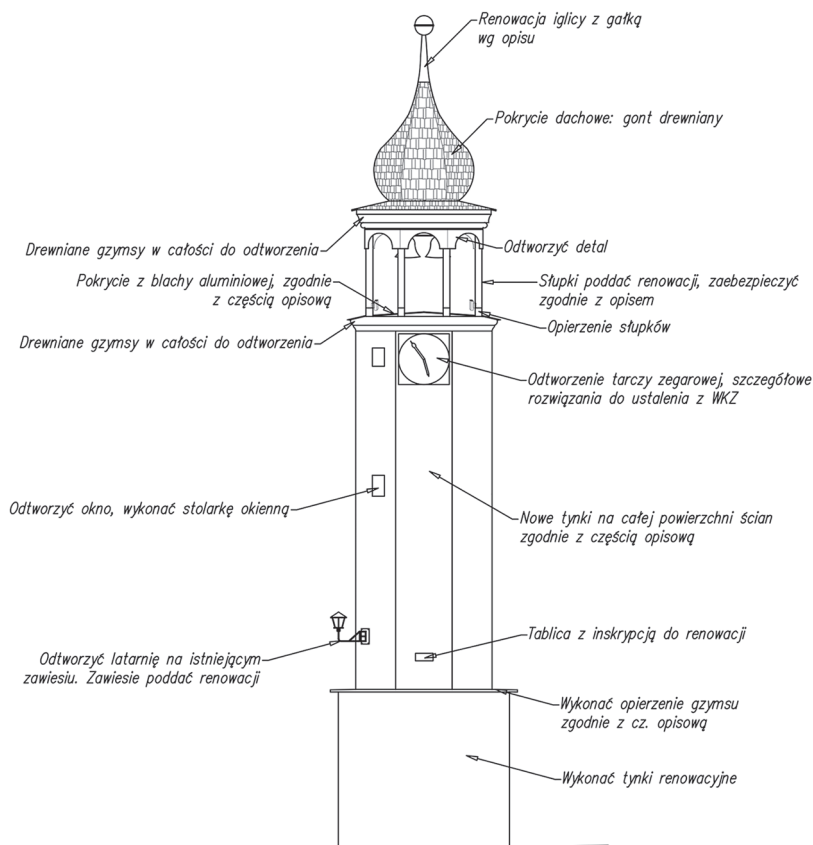
Rysunek z projektu budowlanego pt. „Rewitalizacja wieży zegarowej na Wzgórzu św. Jerzego”
